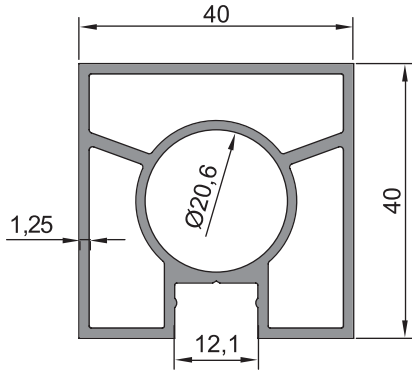
08 - 075 (0,862 kg/m)
