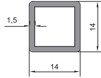
08 - 060 (0,201 kg/m)
