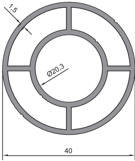
08 - 070 (0,897 kg/m)
