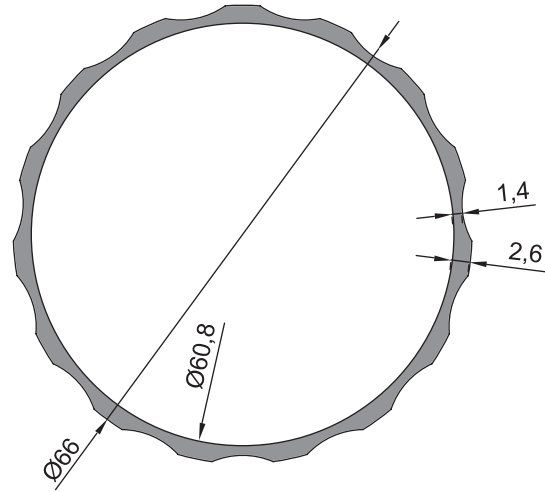
08 - 017 (1,115 kg/m)
