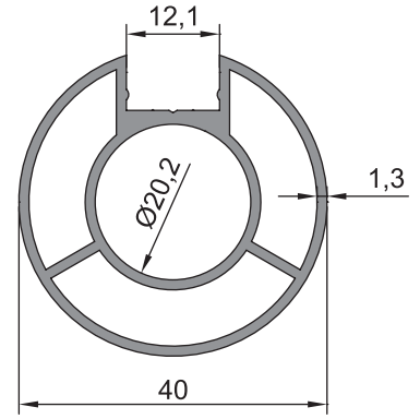
08 - 016 (0,768 kg/m)
