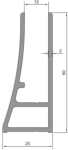
08 - 059 (0,894 kg/m)
