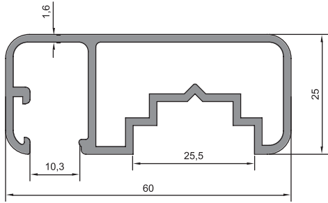
08 - 056 (0,867 kg/m)
