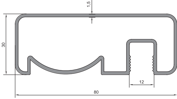
08 - 054 (1,073 kg/m)
