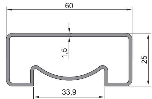
08 - 043 (0,722 kg/m)
