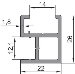
08 - 025 (0,464 kg/m)
