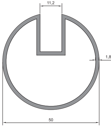
08 - 061 (0,924 kg/m)
