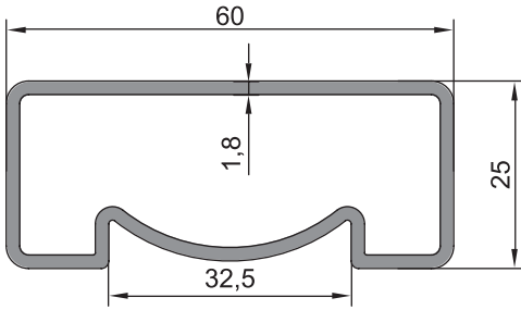
08 - 022 (0,845 kg/m)
