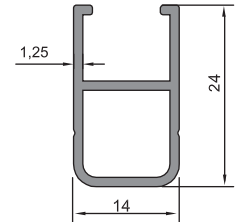
08-124 (0,241 kg/m)
