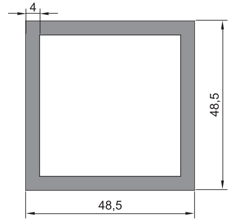
08 - 029 (1,930 kg/m)
