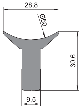
08 - 034 (0,853 kg/m)
