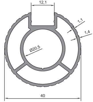
08 - 067 (0,805 kg/m)
