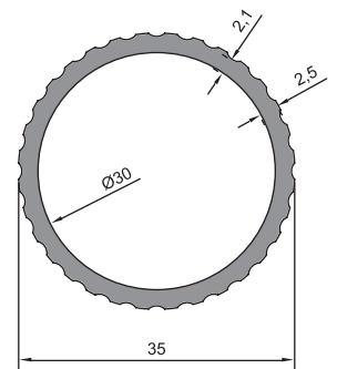
08 - 065 (0,640 kg/m)
