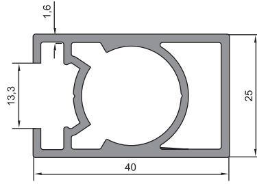
08 - 053 (0,778 kg/m)
