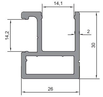
08 - 058 (0,623 kg/m)
