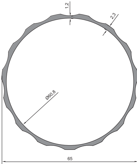
08 - 047 (0,970 kg/m)
