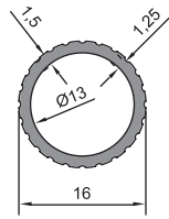
08 - 066 (0,176 kg/m)
