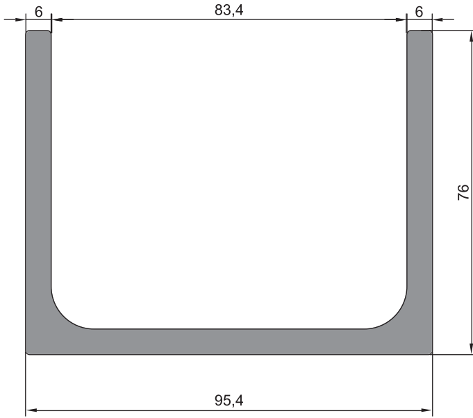
08 - 032 (3,940 kg/m)
