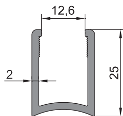
08 - 002 (0,355 kg/m)
