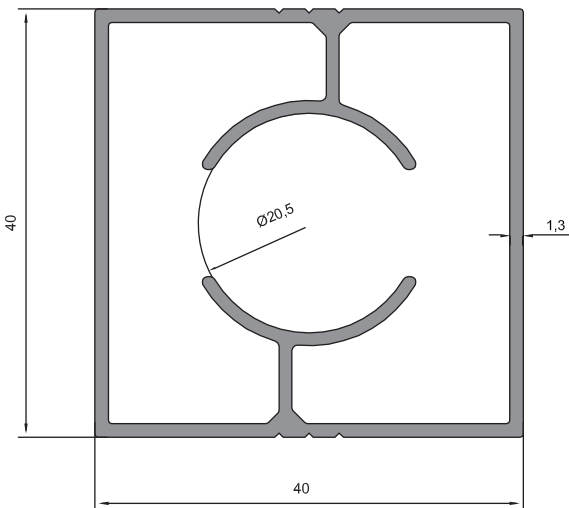
08 - 123 (0,753kg/m)
