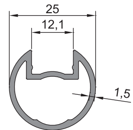
08 - 003 (0,352 kg/m)
